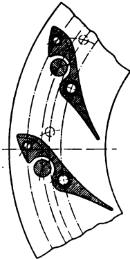
Fig. 32. Schnitt durch die Leitfschaukeln.
